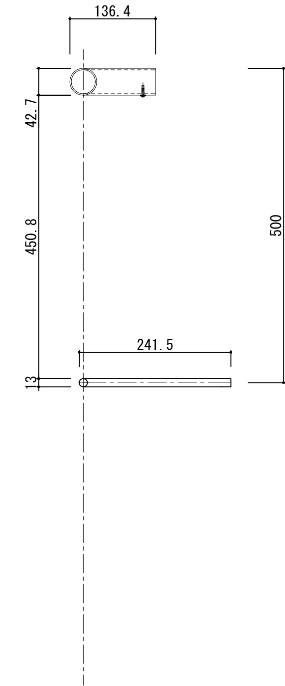
B矢視図
