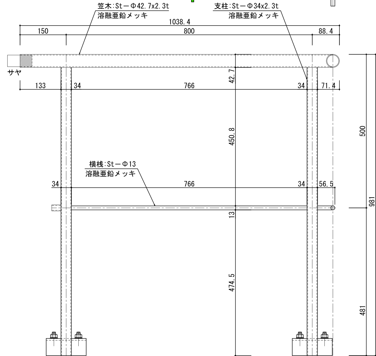
A矢視図
