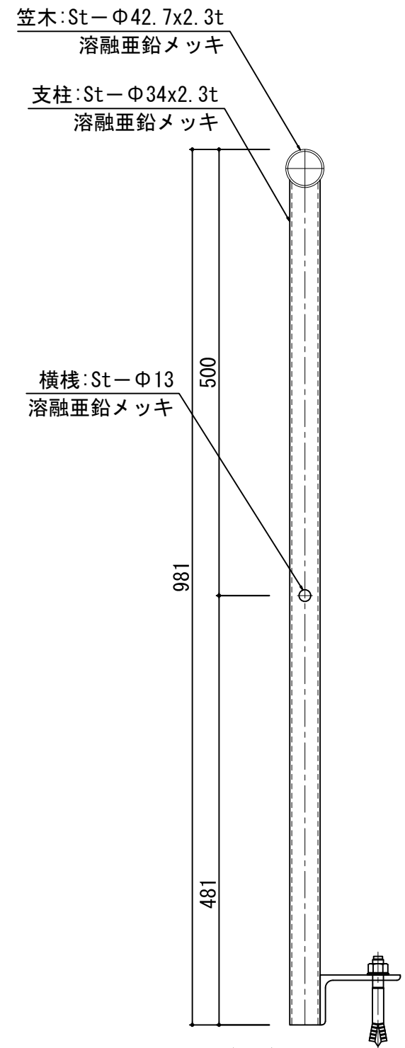
A矢視図
