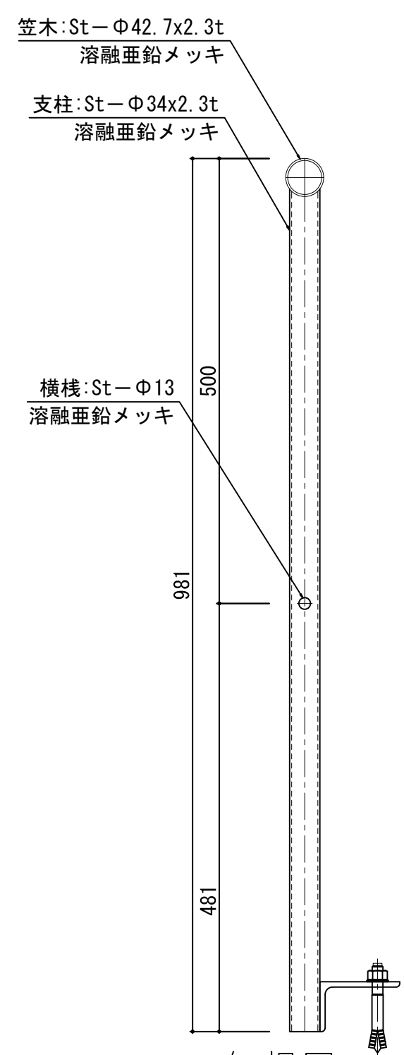
ア矢视图
