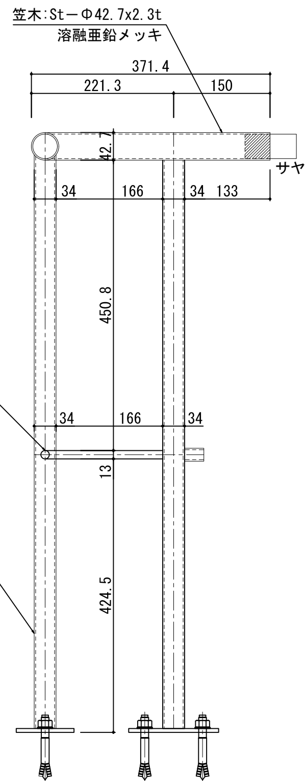
B矢視図
