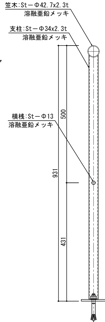
ア矢視図
