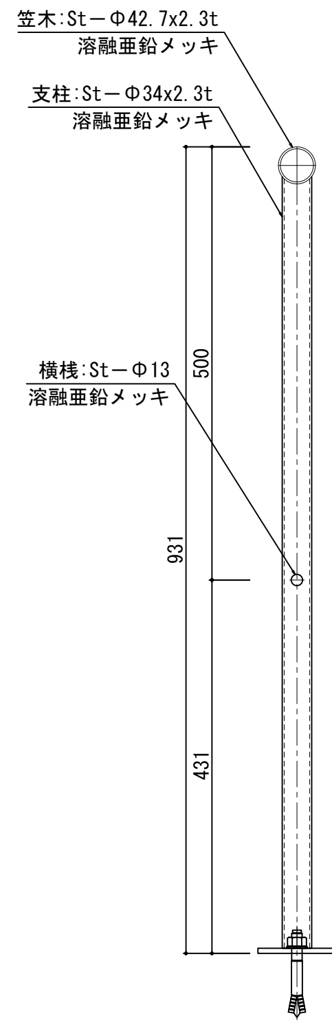
ア 矢視図
