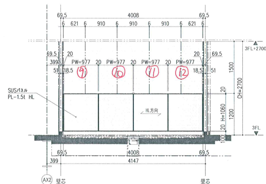
4 矢視 立面図 (S=1/30)
