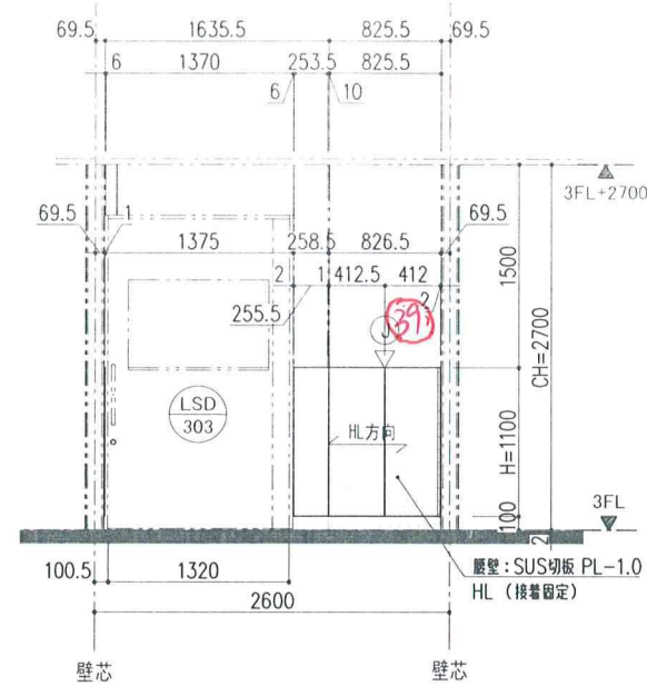
22 矢視 立面図 (S=1/30)
