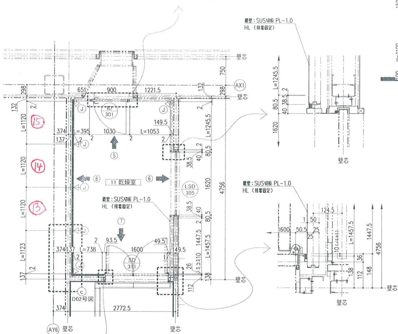
B部 平面図(S=1/30) 11 乾燥室
