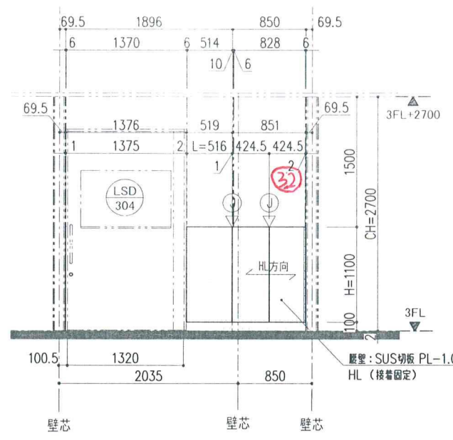
18A 矢視 立面図 (S=1/30)
