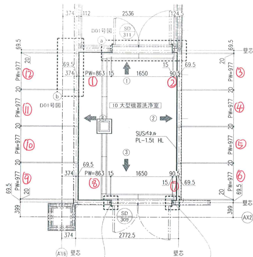
A 平面図 (S=1/30) 10 大型機器洗浄室
