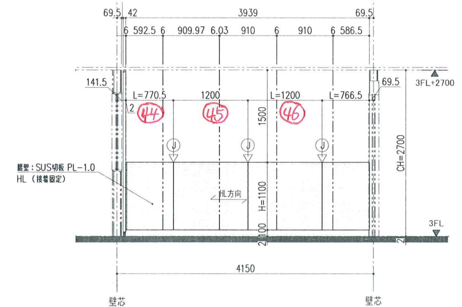
25 矢視 立面図 (S=1/30)
