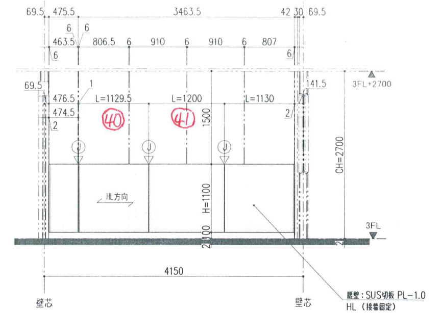
23 矢視 立面図 (S=1/30)
