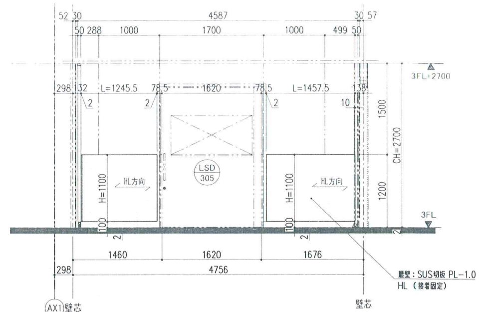
6 矢視 立面図(S=1/30)
