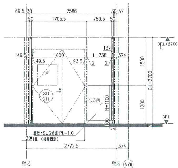
7 矢視 立面図(S=1/30)
