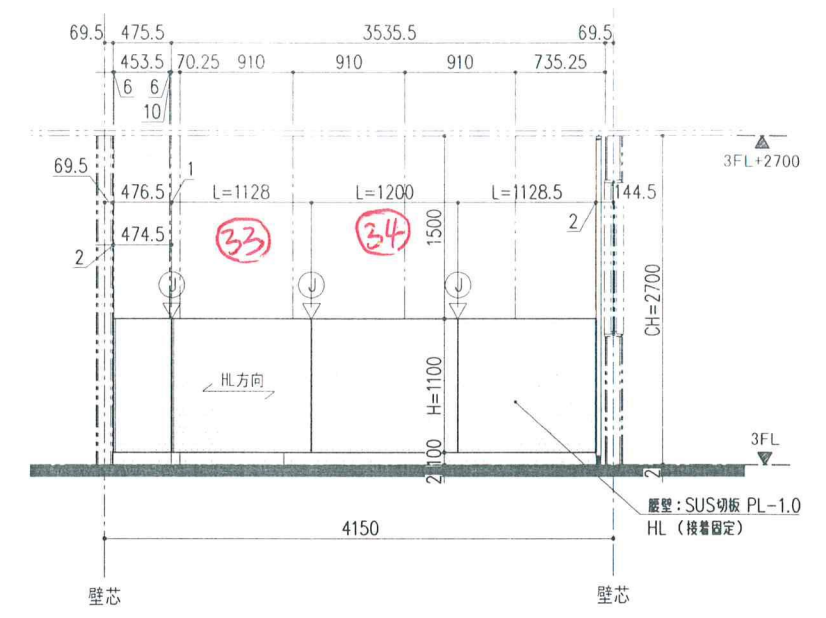
19 矢視 立面図 (S=1/30)
