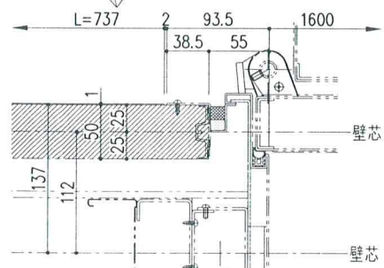
B部 平面図(S=1/30) 11 乾燥室
