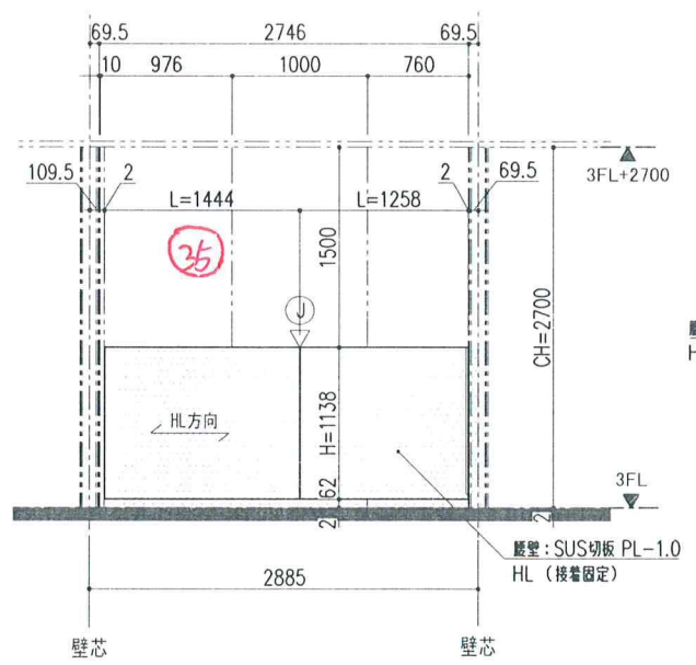
20 矢視 立面図 (S=1/30)
