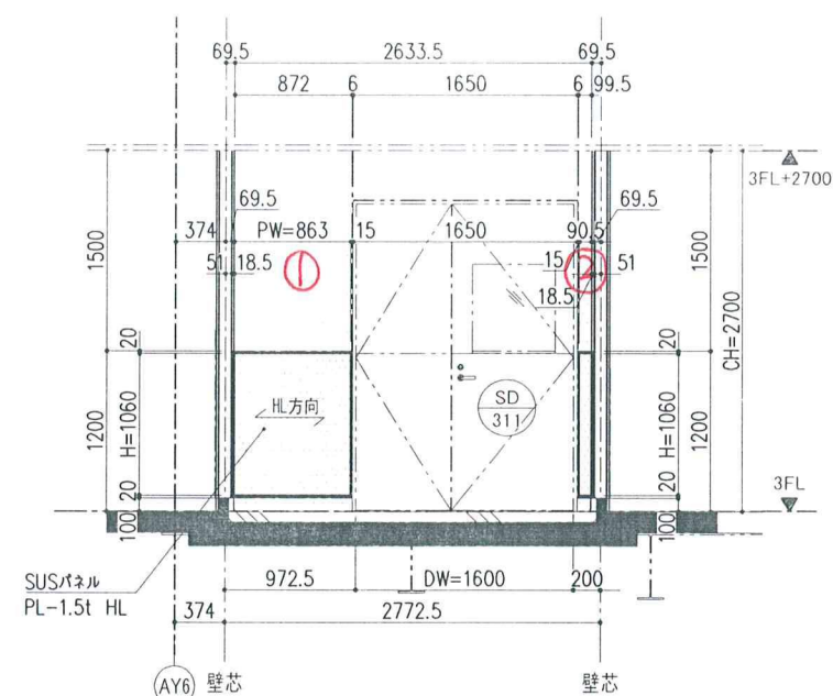
1 矢視 立面図 (S=1/30)
