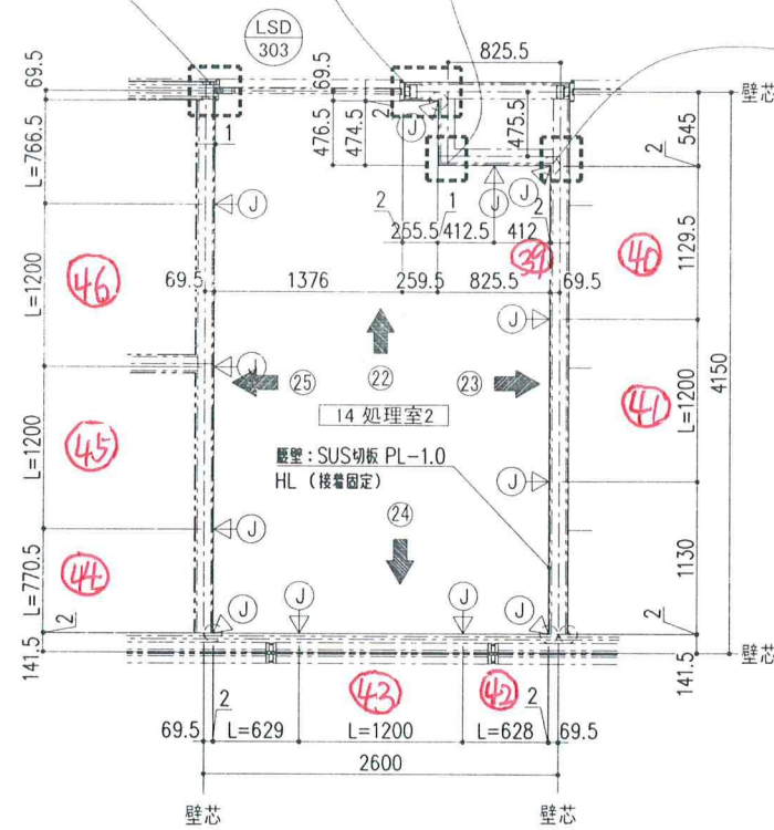
F部 平面図 (S=1/30)
