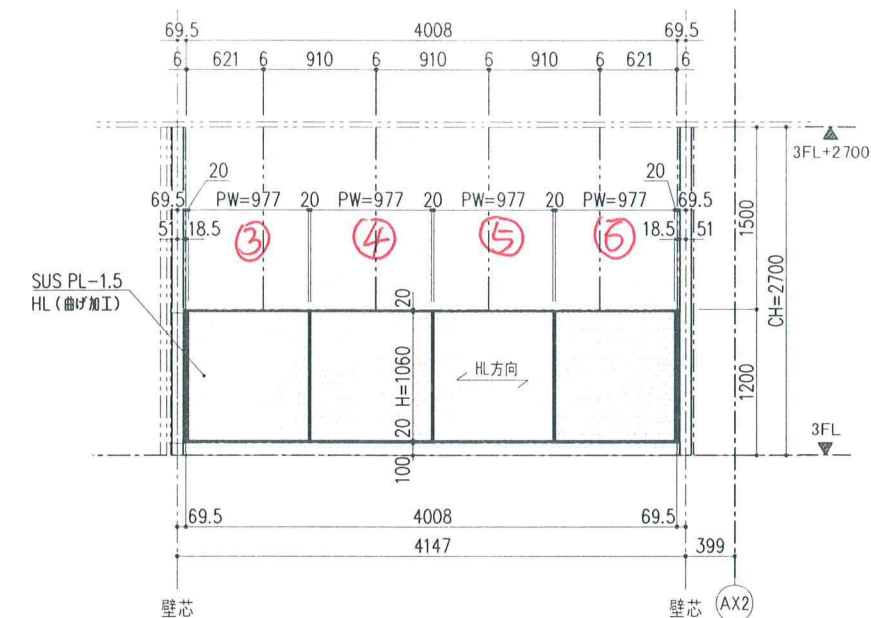
2 矢視 立面図 (S=1/30)
