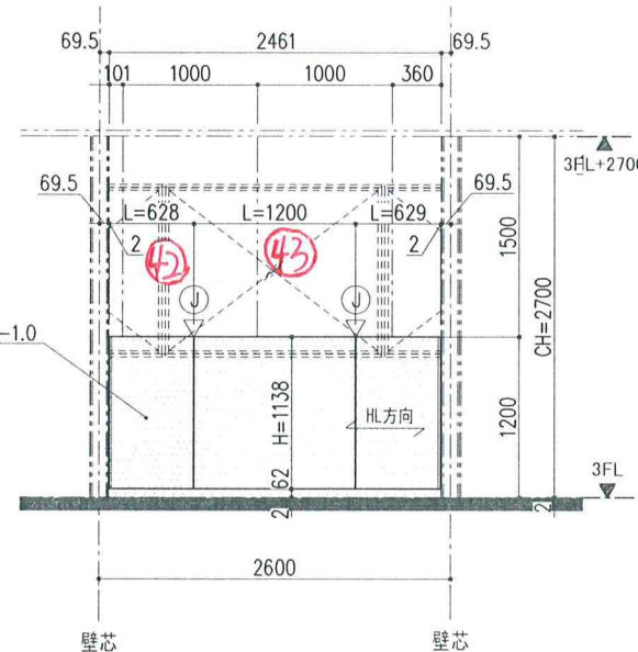
24 矢視 立面図 (S=1/30)
