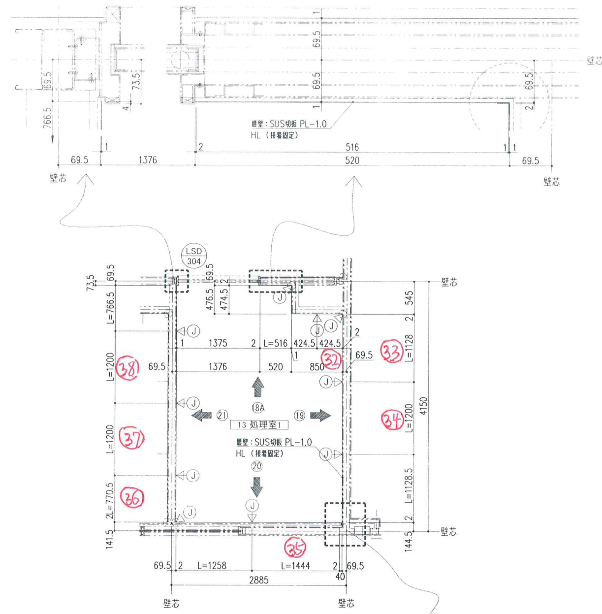
E部 平面図 (S=1/30) 13 処理室1
