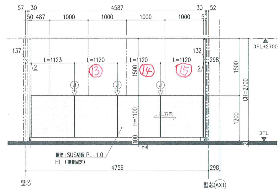
8 矢視 立面図(S=1/30)
