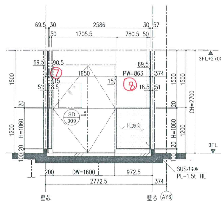
3 矢視 立面図 (S=1/30)
