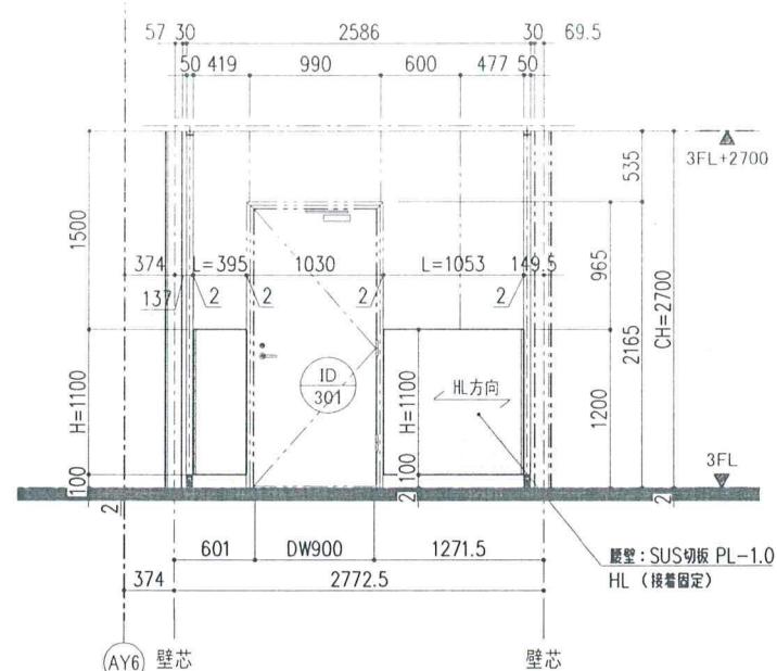
5 矢視 立面図(S=1/30)
