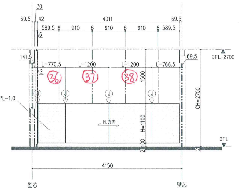
21 矢視 立面図 (S=1/30)
